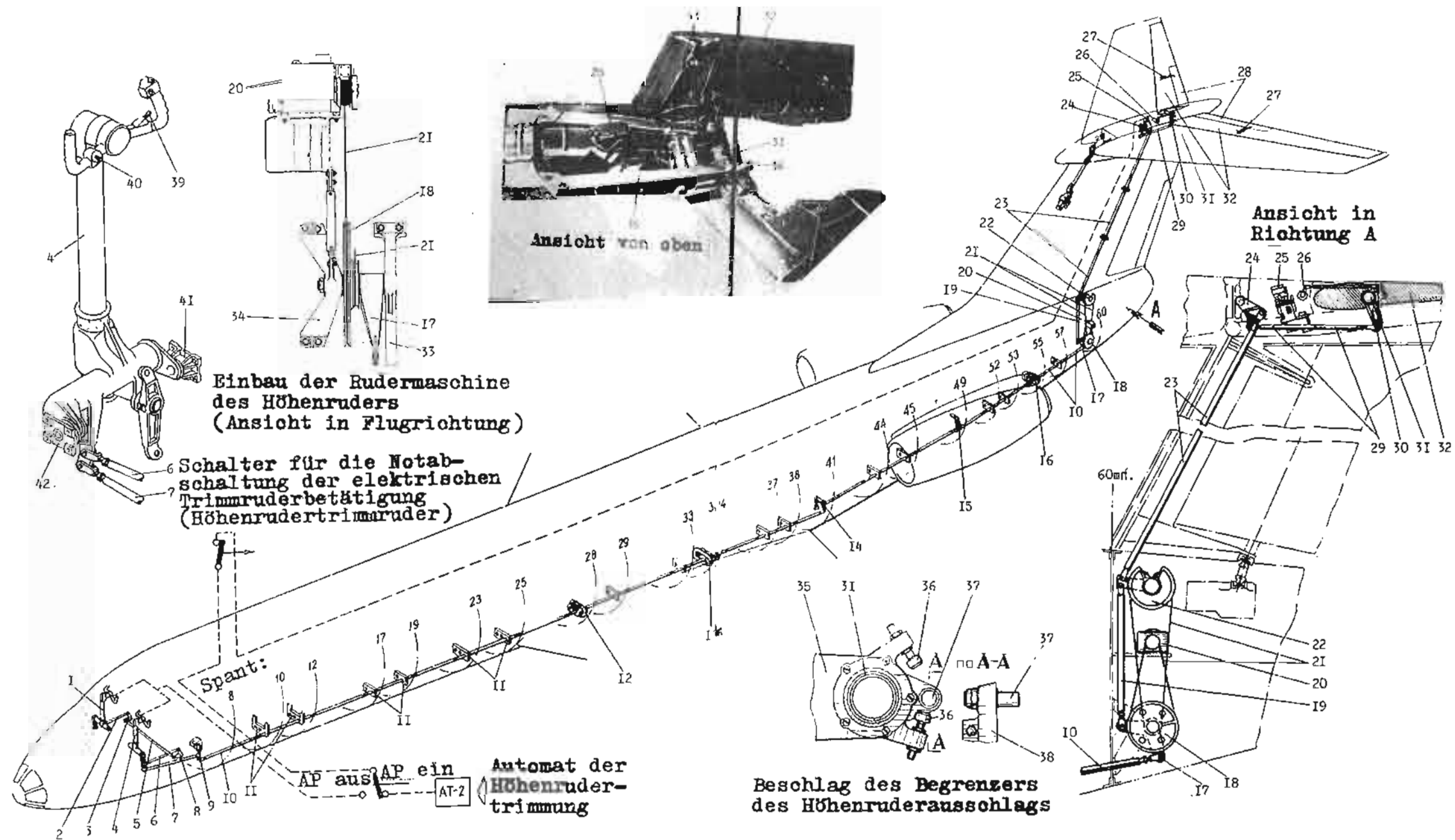
Abb. 42 Schema der Höhenrundersteuerung
