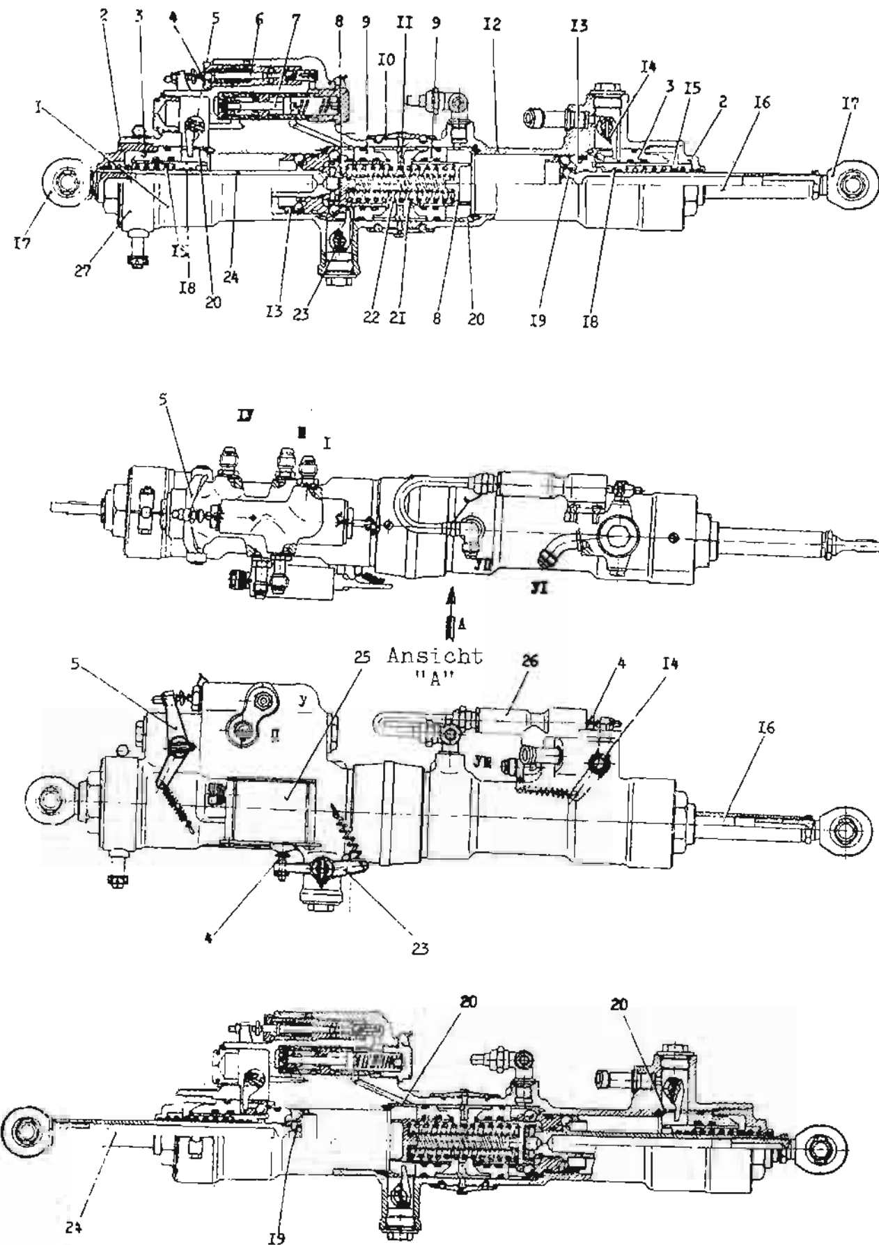
Abb. 112 Hydraulikzylinder des Betätigungsmechanismus der hinteren Hauptfahrwerksklappen
