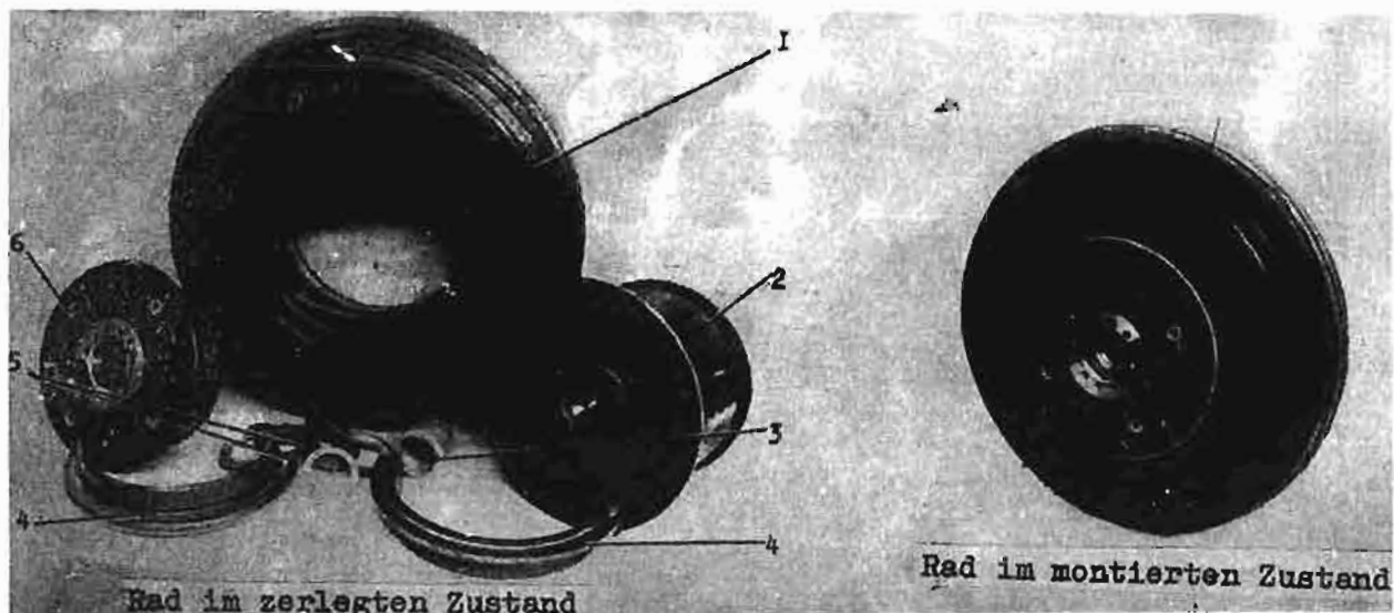
Abb. 107 Bremsrad KT-113 mit Hochdruckreifen 930 x 304W
