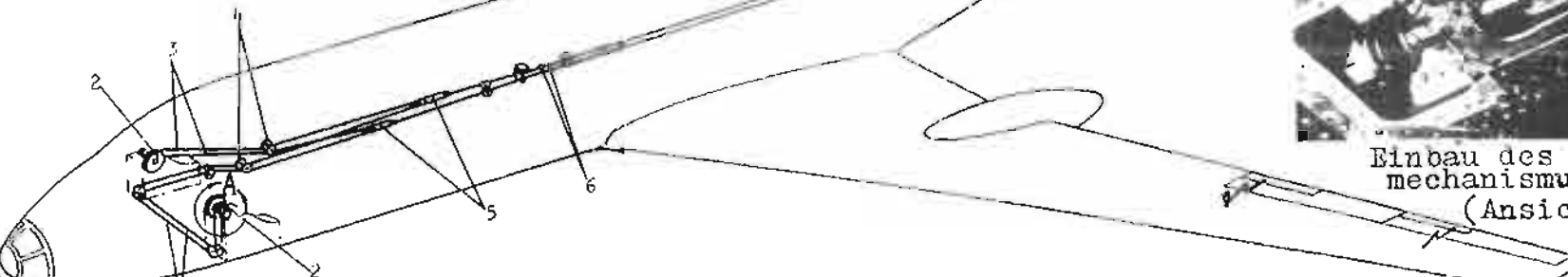
Abb. 43 Schema der mechanischen Höhenrudertrimmerbetätigung
