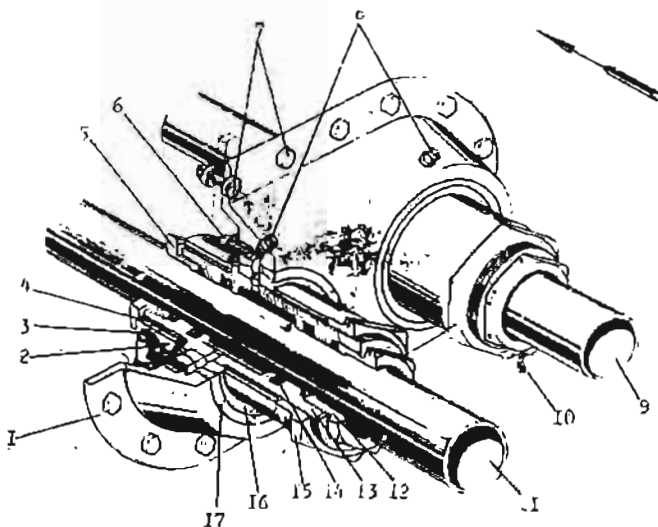
Abb. 41 Druckdichte Durchführung
