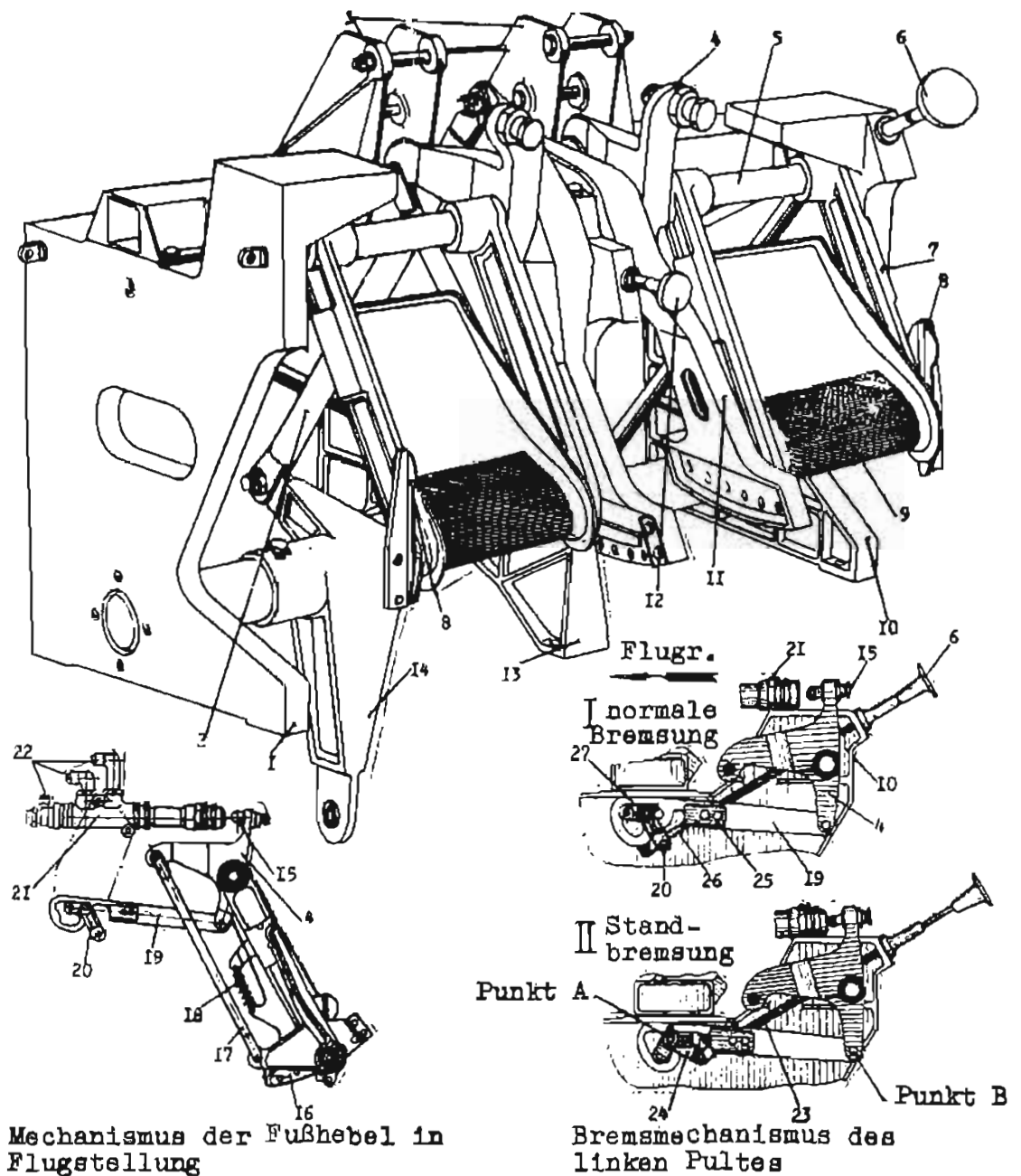
Abb. 47 Das Pedalpult des 1. Piloten
