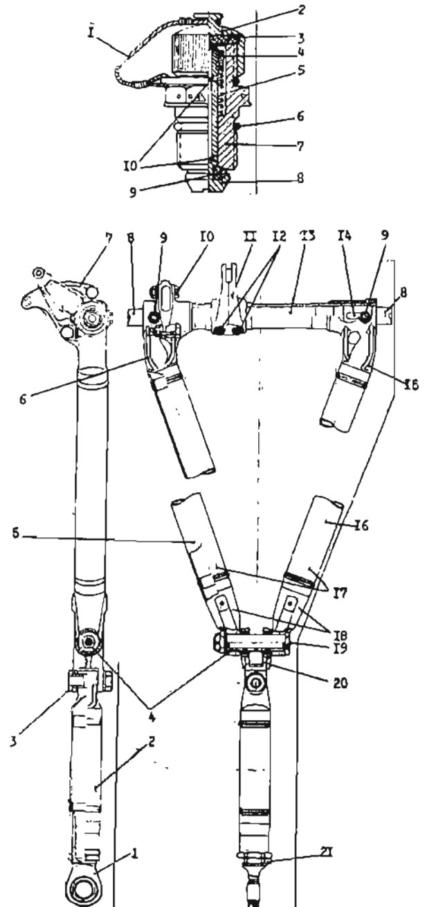
Abb. 88 Knickstrebe des Bugfahrwerkes
