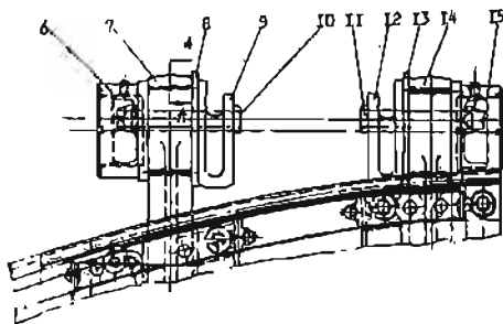
Ansicht A
