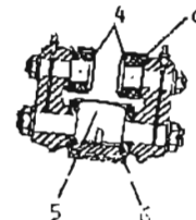
Wagen der inneren Landeklappe
