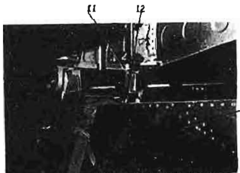
hintere Befestigung der Höhenflosse
