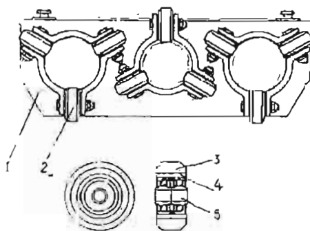
Abb. 40 Rollenführungen
