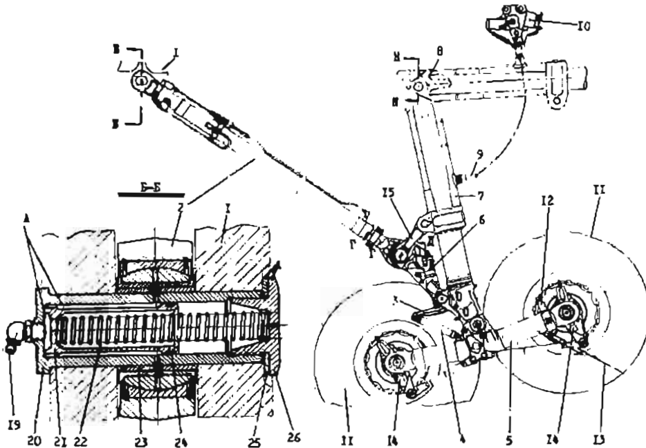
Aufhängung d. Arb. Zyl. an der Tragfläche
