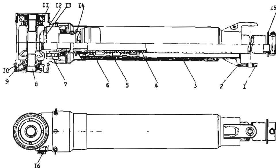
Abb. 76 Rumpflappenspindel 124 A-5701-210
