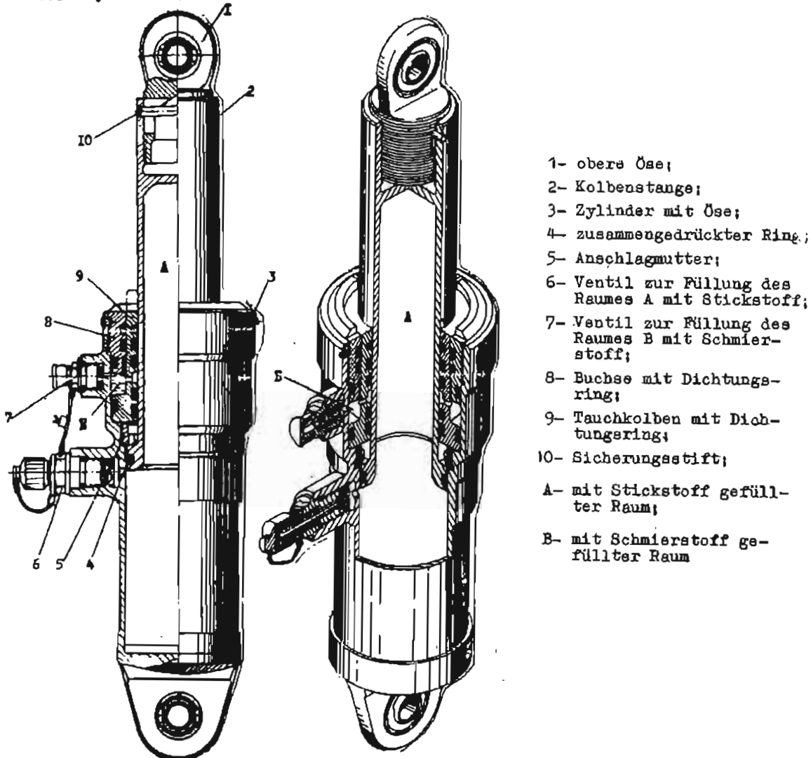
Abb. 103 Stabilisierungsdämpfer
