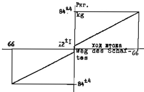
Abb. 31 Federbelastung der Querruder
