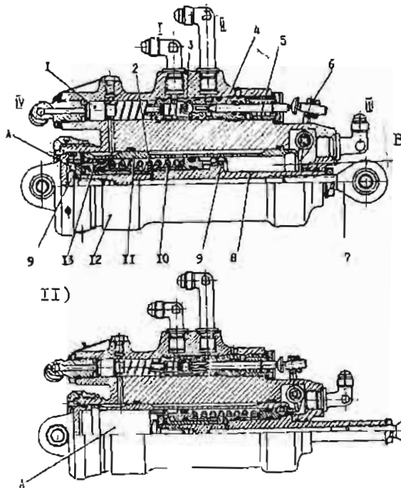
Abb. 96 Betätigungszyylinder der hinteren Bugfahrwerksklappen in zwei Stellungen
