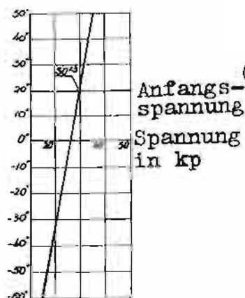
Abhängigkeit der Seilspannung in der Steuerungsanlage der Höhenrudertrimmruder von der Temperatur
