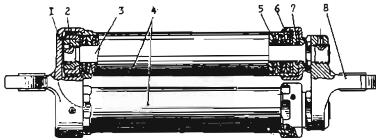
Abb. 104 Federzugstange des Schwenkmechanismus des Fahrwerkswagens
