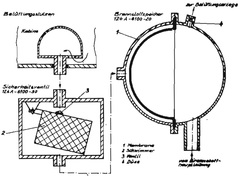
Abb. 142 Kraftstoffspeicher, Sicherheitsventil und Belüftungszulzen (Schema)
