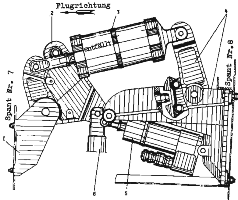
Abb. 49 Einbau des Flugbelästers (Draufsicht) 1 - Halterung; 2 - dreiarmliger Schwinghebel; 3 - Flugbelaster; 4 - Einschaltmechanismus; 5 - Elt-Antrieb MP-100M-16; 6 - Steuerstange (zum 1. Piloten).
