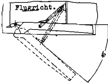
Aufhängung des Landeschildes
