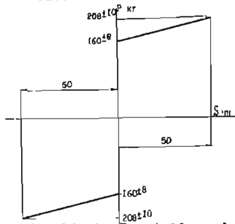
Graphische Darstellung der Arbeit des Bahnbelasters
