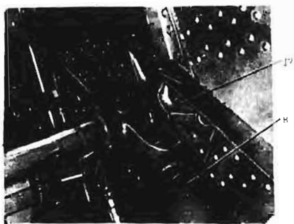
Rechter Beschlag zur Befestigung der Knickstrebe am Längsträger (Ansicht von unten in Flugrichtg.)
